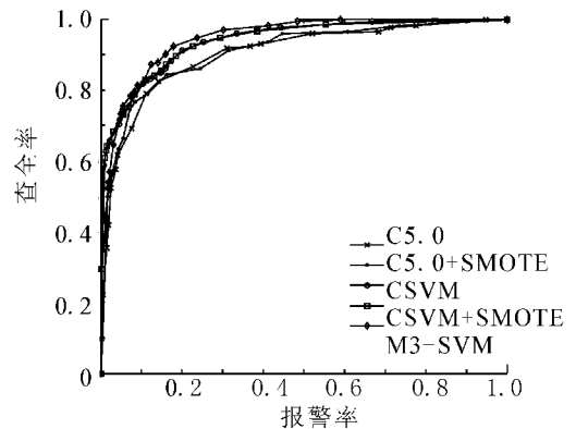
图 1 Park 数据的 ROC 曲线
